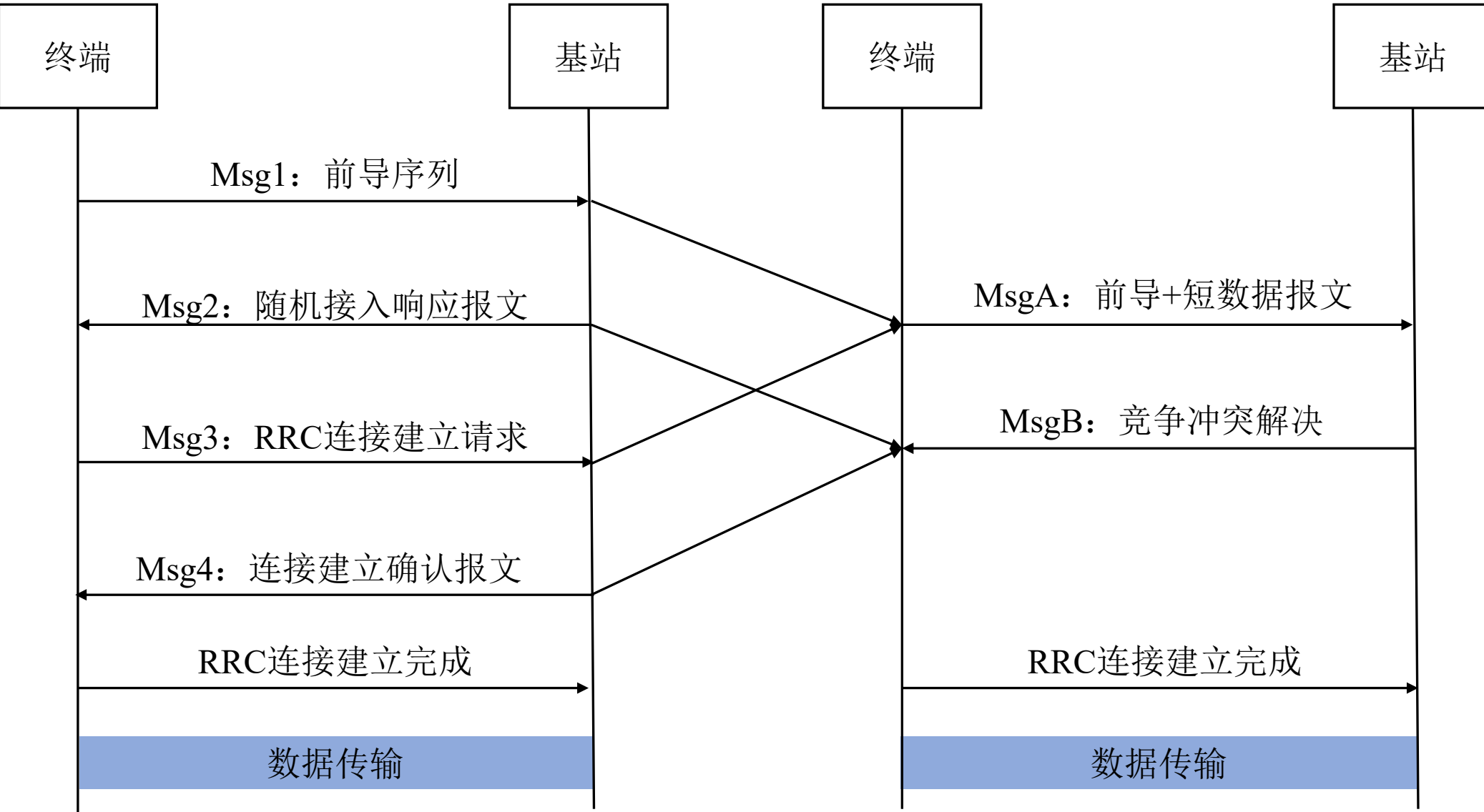
基于连接的四步随机接入过程
